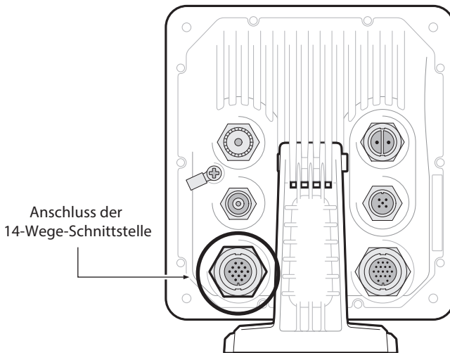
Abbildung 12 Anschluss der seriellen Dateneingangsportes
