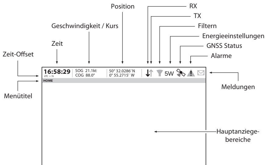
Abbildung 22 Display-Layout
