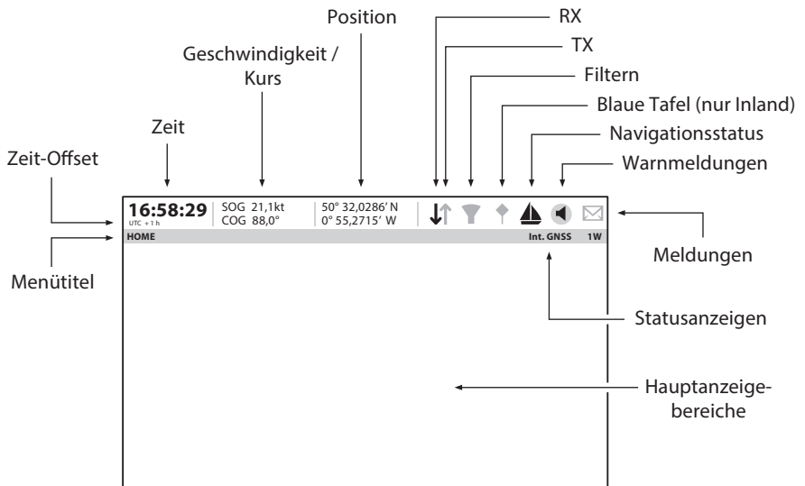
Abbildung 21 Display-Layout
