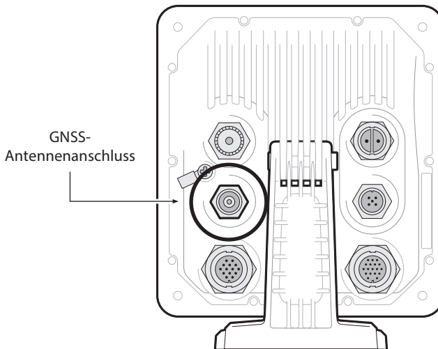
Abbildung 7 Position der GNSS-Antenne
