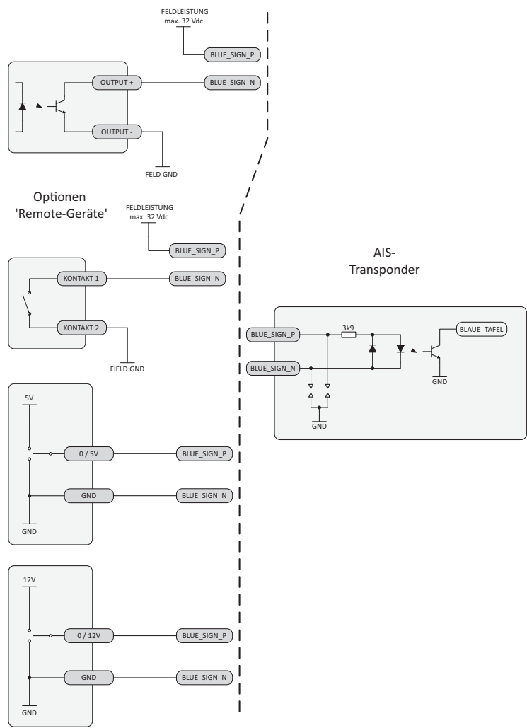
Abbildung 28 Anschlussoptionen für die 'Blaue Tafel'-Schnittstelle
