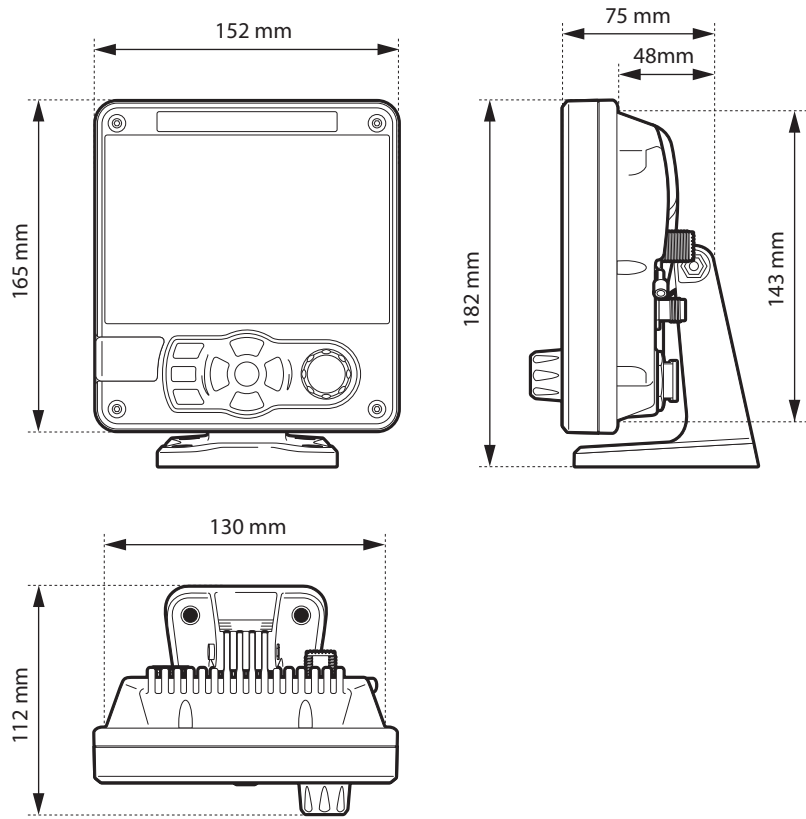
Abbildung 31 Abmessungen des Transponders
