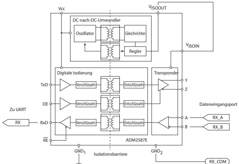
Abbildung 29 Schema des Eingangsports
