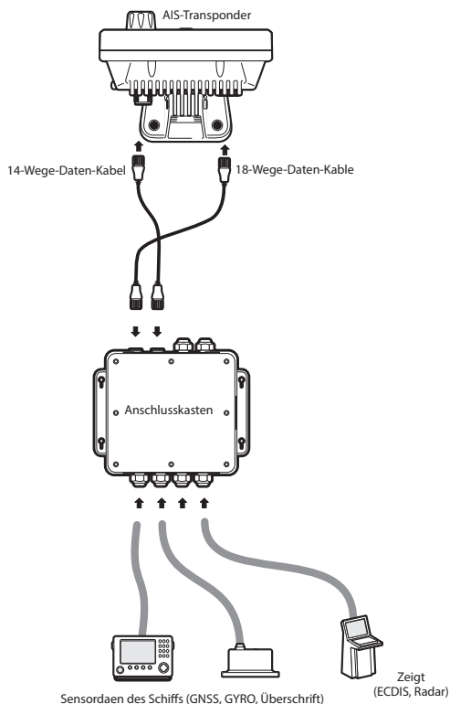
Abbildung 35 Anschluss externer Geräte
