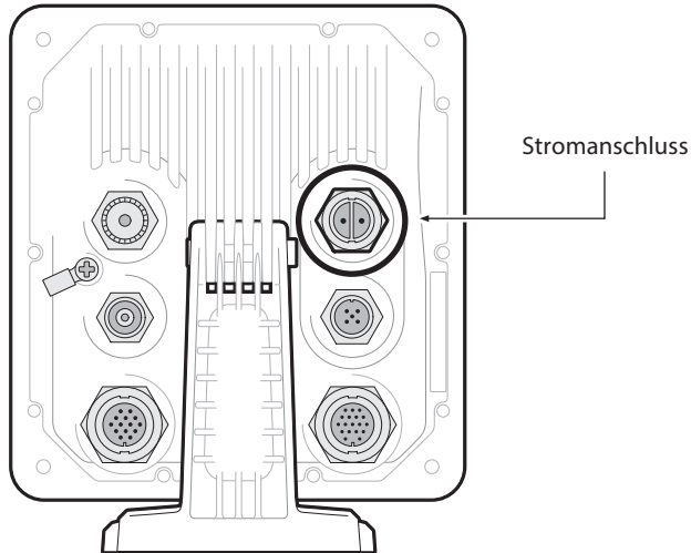
Abbildung 15 Stromanschluss
