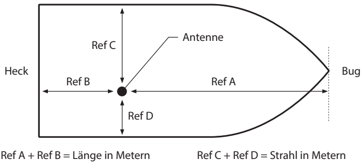
Abbildung 23 Messen der Abmessungen des Schiffs
