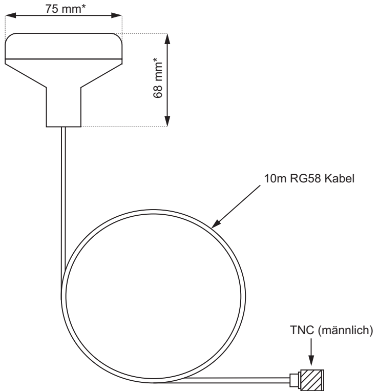
Abbildung 32 GNSS-Antenne
