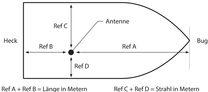
Abbildung 36 GNSS-Antennenposition
