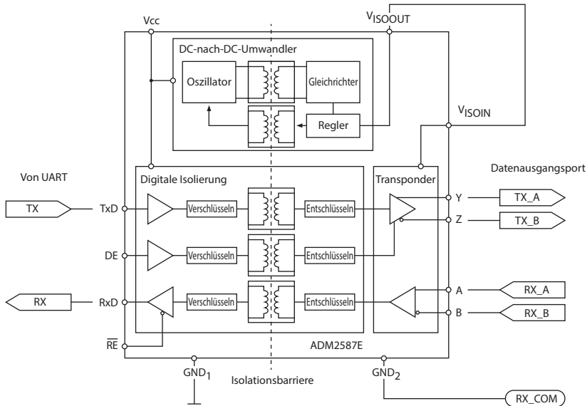
Abbildung 30 Schema des Datenausgangsports
