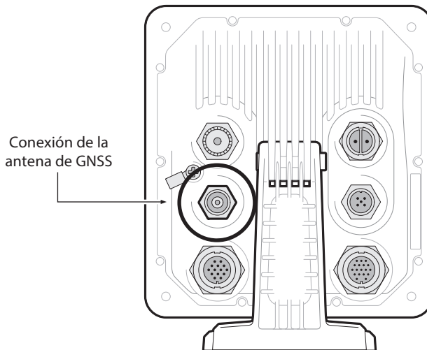
Figura 7 Ubicación de la antena de GNSS
