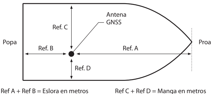
Figura 23 Medición de las dimensiones de la embarcación
