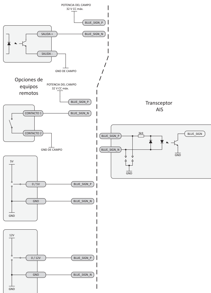
Figura 28 Opciones de conexión de la interfaz de señal azul
