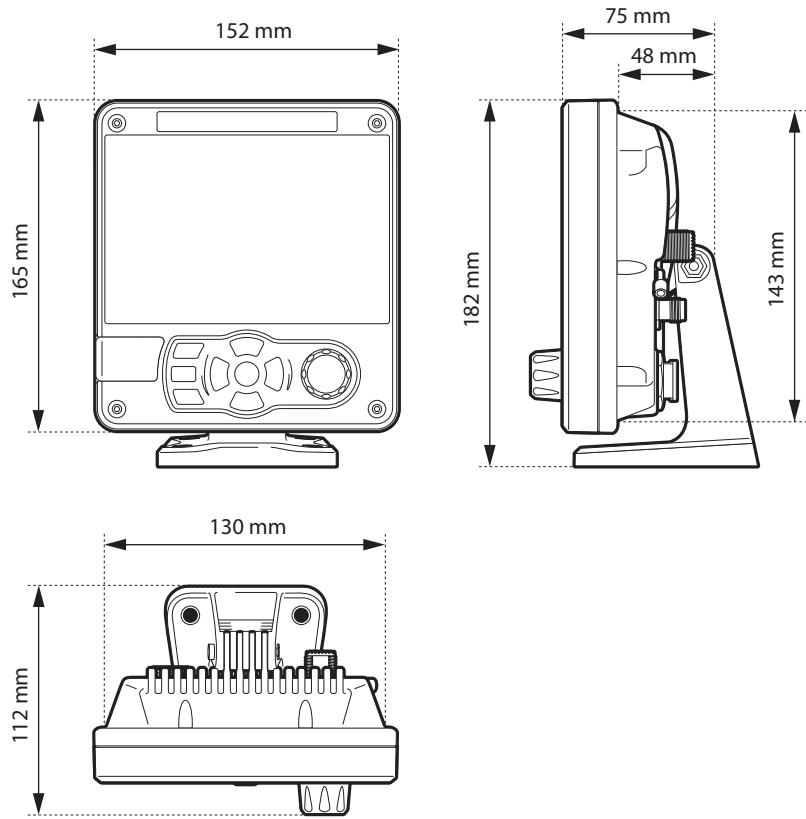
Figura 31 Dimensiones del transceptor AIS
