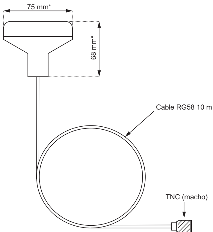
Figura 32 Antena GNSS
