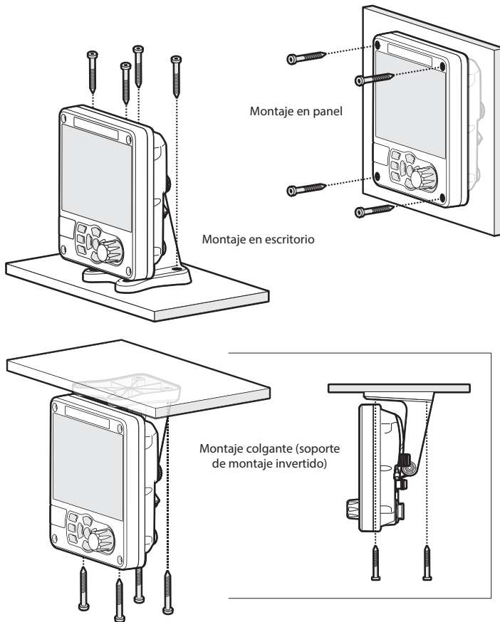
Figura 4 Montaje del transceptor AIS
