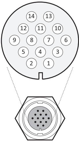
Figura 12 Conexiones del cableado del conector de 14 vías
