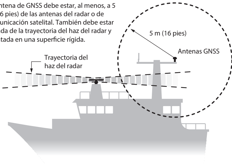
Figura 7 Ubicación de la antena de GNSS
