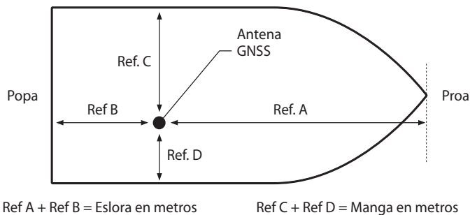
Figura 36 Posición de la antena de GNSS
