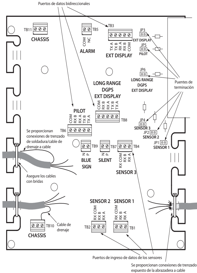
Figura 34 Conexiones de la caja de conexiones
