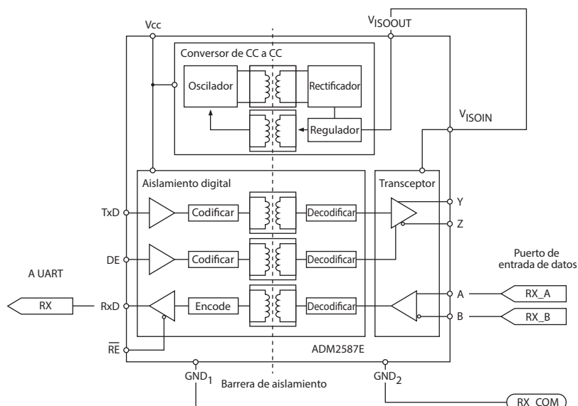
Figura 29 Diagrama del puerto de ingreso
