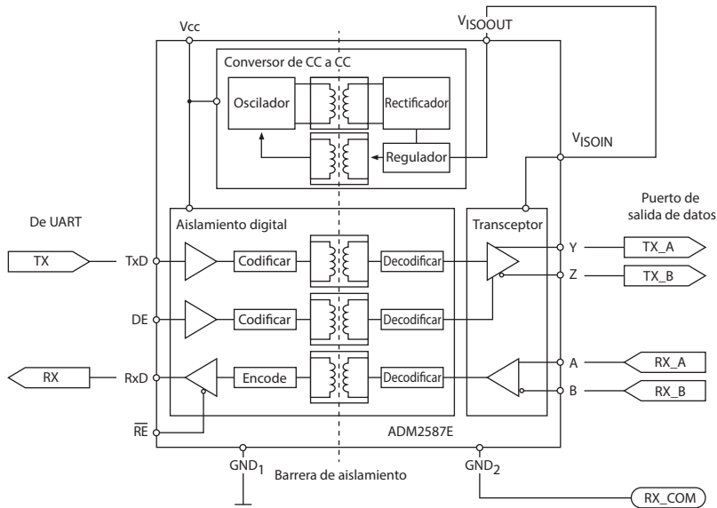
Figura 30 Diagrama del puerto de salida de datos
