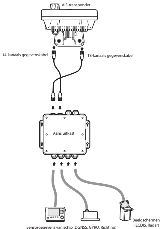
Afbeelding 35 De externe apparatuur aansluiten
