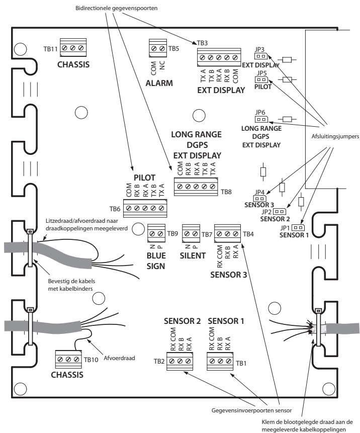
Afbeelding 34 Aansluitingen aansluitkast
