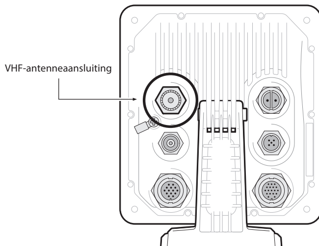
Afbeelding 10 Aansluiting VHF-antenne
