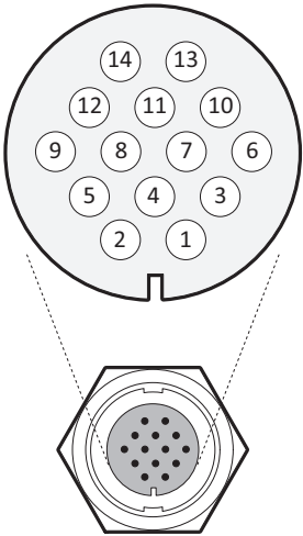
Afbeelding 12 Bedradingsaansluitingen van 14-wegs connector
