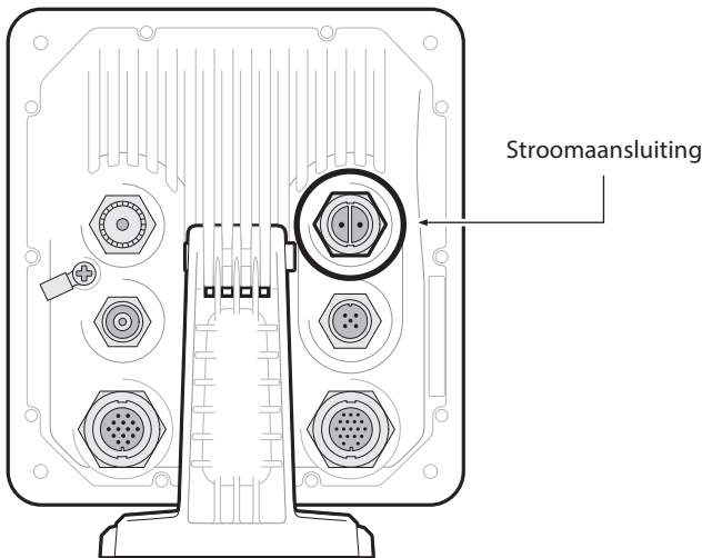
Afbeelding 15 Stroomaansluiting
