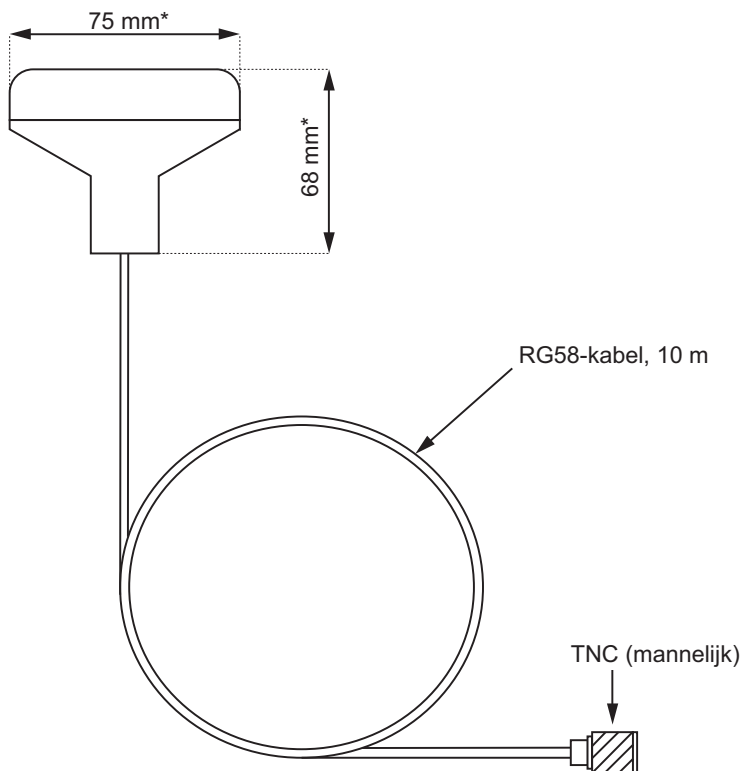
Afbeelding 32 GNSS-antenne
