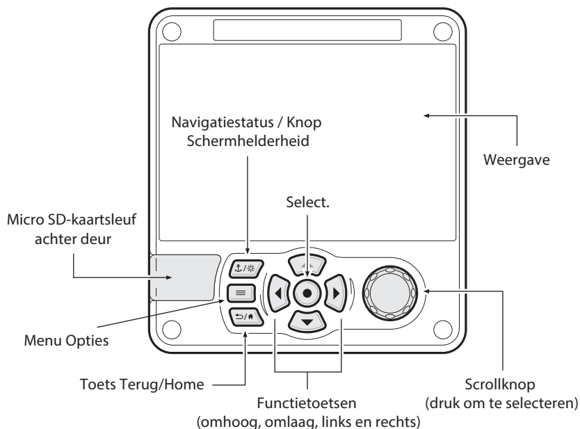
Afbeelding 18 Voorpaneel van AIS-transponder
