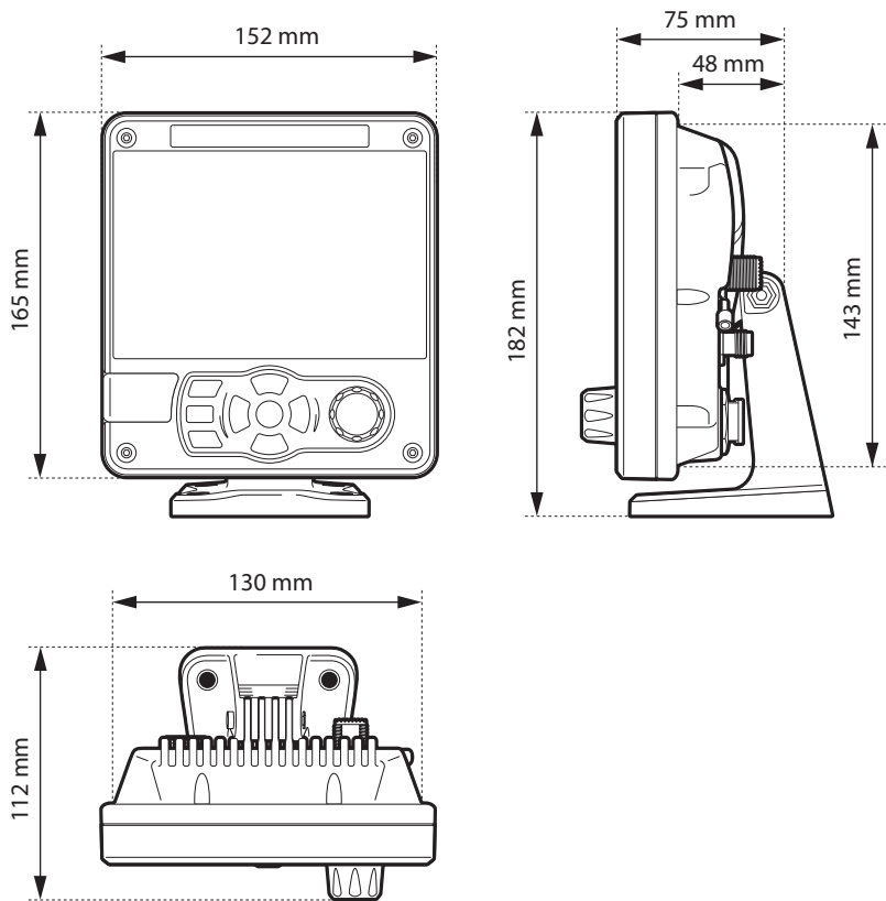
Afbeelding 31 Afmetingen van AIS-transponder
