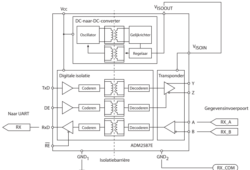
Afbeelding 29 Schema ingangspoort
