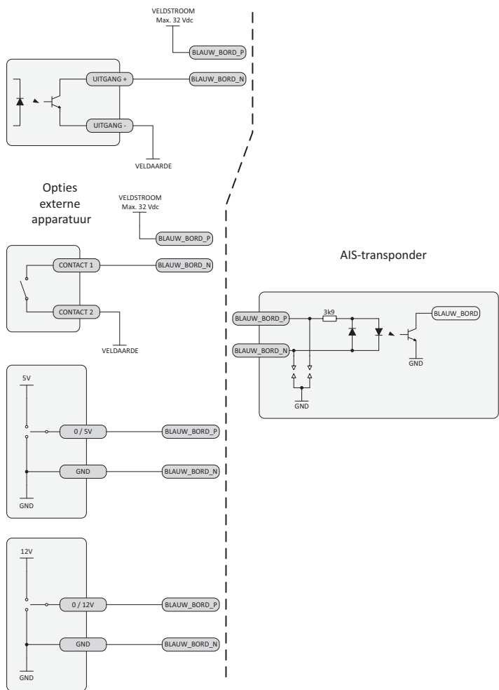
Afbeelding 28 Aansluitmogelijkheden voor 'blauw bord'-interface
