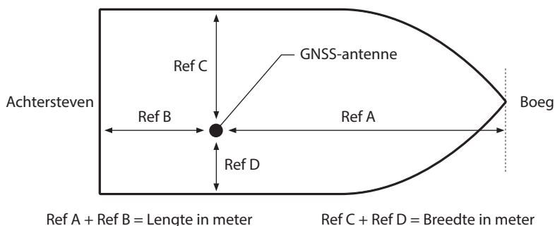
Afbeelding 23 Afmetingen van schip
