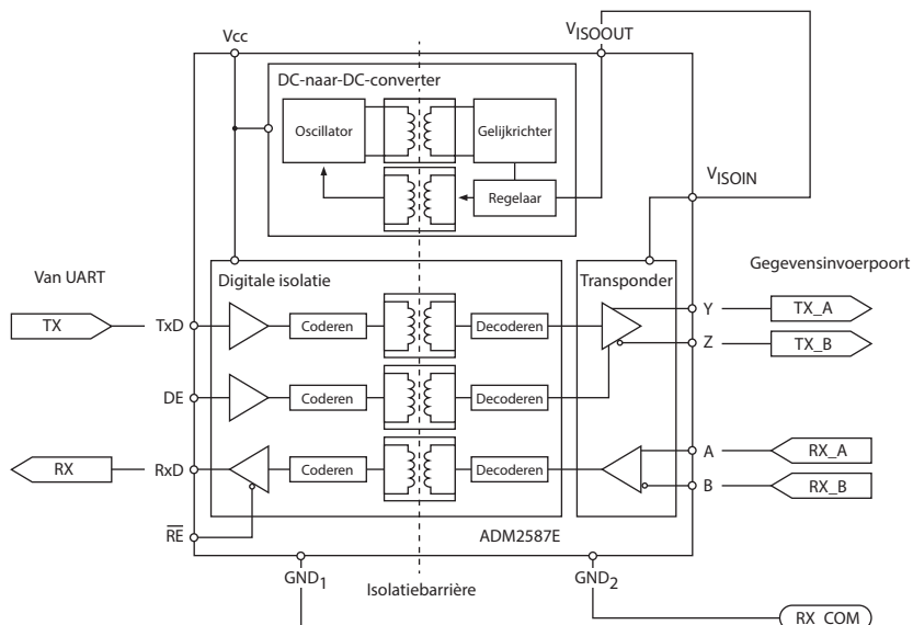
Afbeelding 30 Schema gegevensuitvoerpoort
