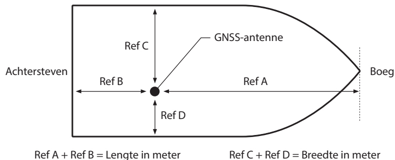
Afbeelding 36 GNSS-antennepositie
